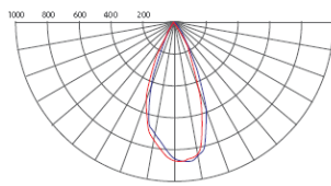
Lichtverteilung
